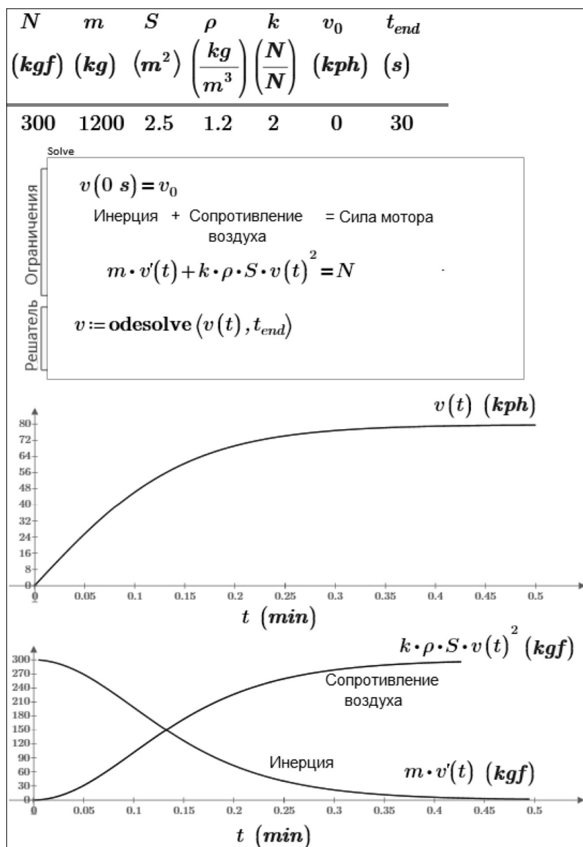
Рис. 7. Задача о старте автомобиля
