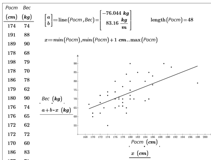
Рис. 3. Сглаживание точек в среде Mathcad
