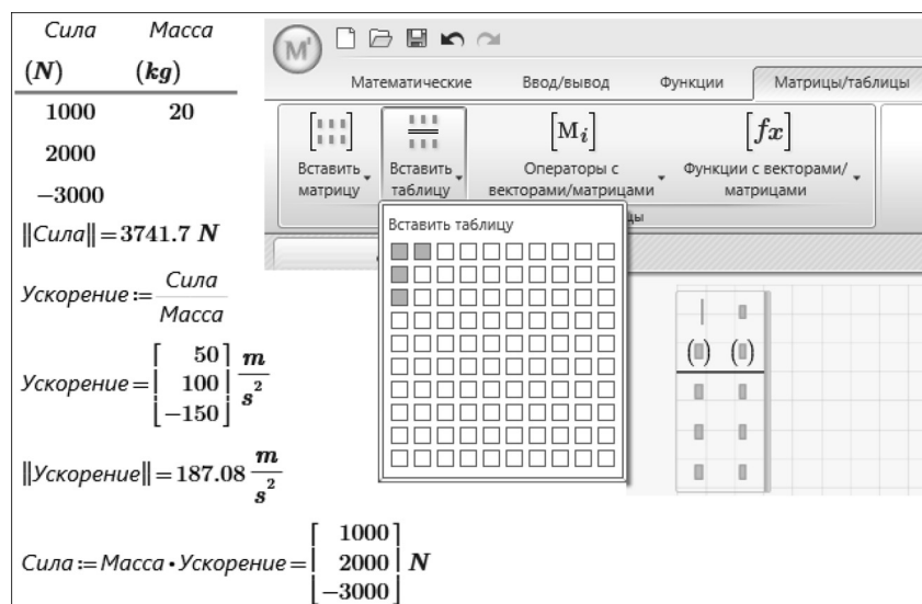
Рис. 1. Задача о движении тела в пространстве (Mathcad Prime)
