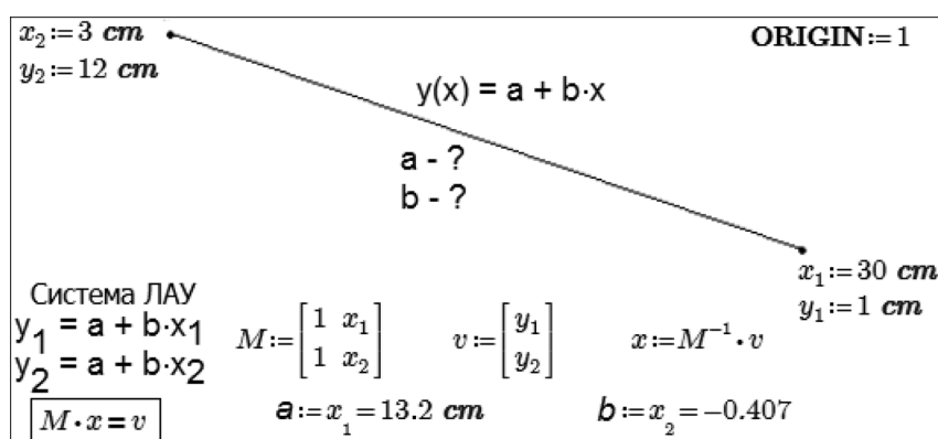
Рис. 4. Задача об уравнении прямой линии
