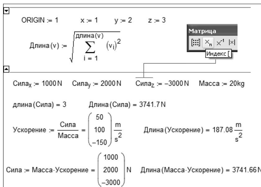
Рис. 2. Задача о движении тела в пространстве (Mathcad 15)
